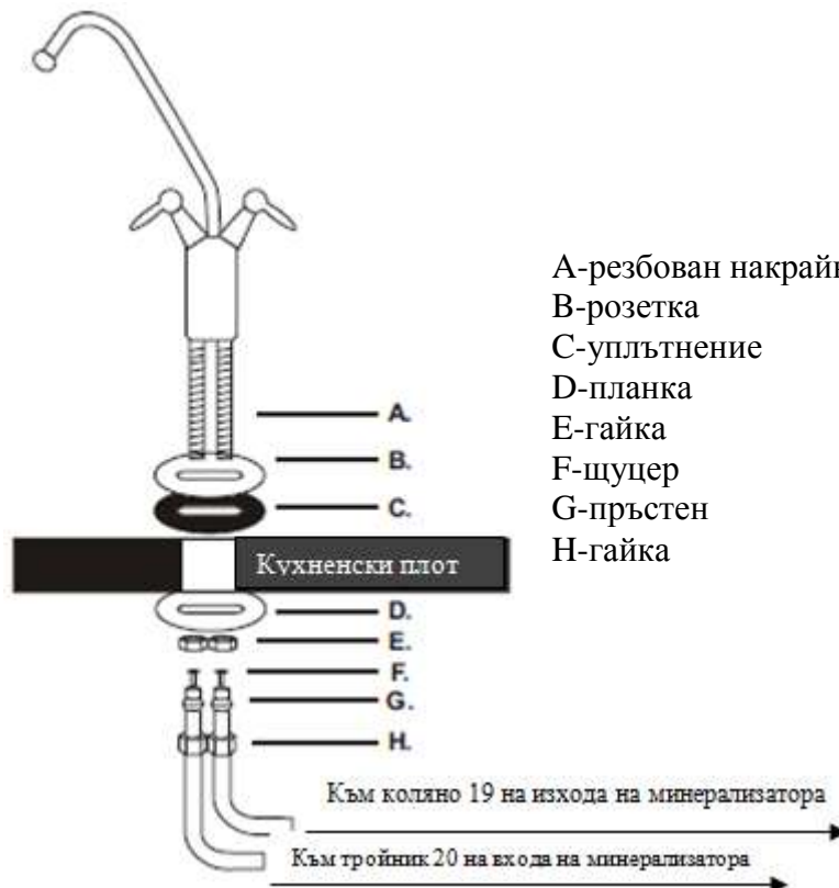
Схема за монтаж на чешмичката
